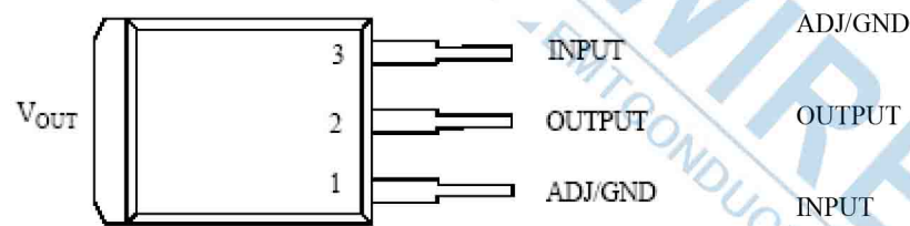
B Package (TO-263)
